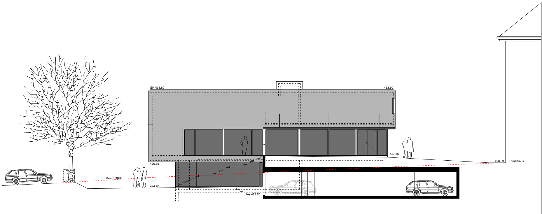
WESTFASSADE
