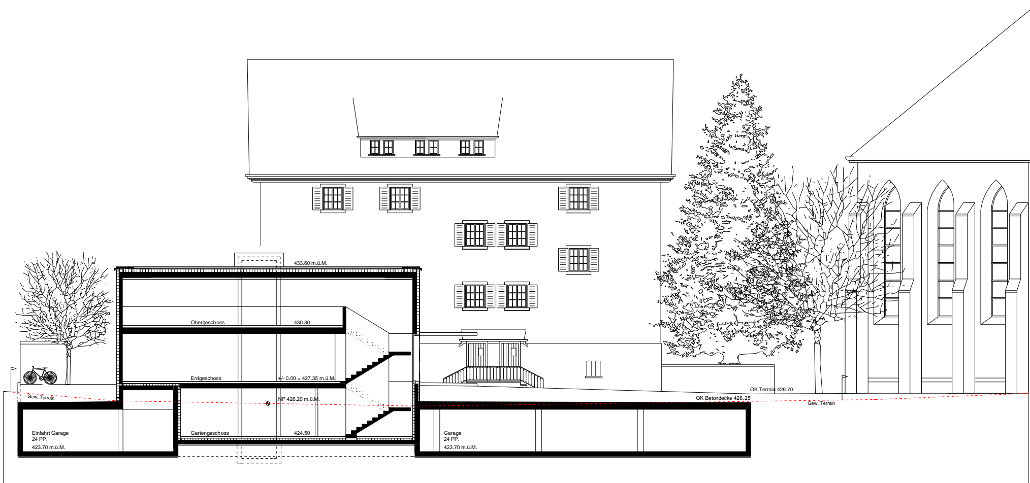
QUERSCHNITT
