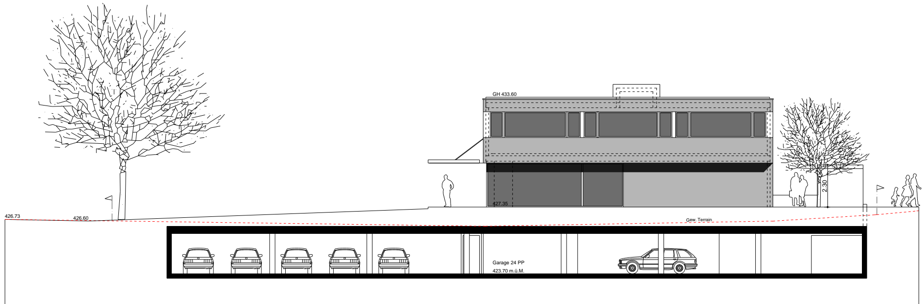
SÜDFASSADE
